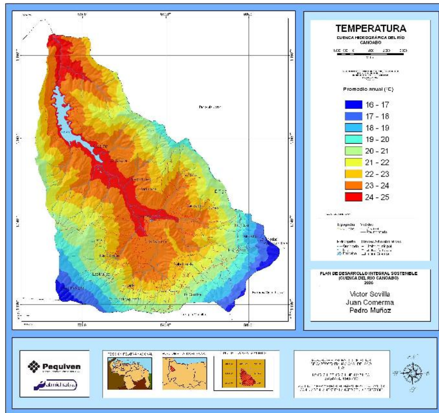
FIGURA 3. Modelo digital de temperatura media anual.
