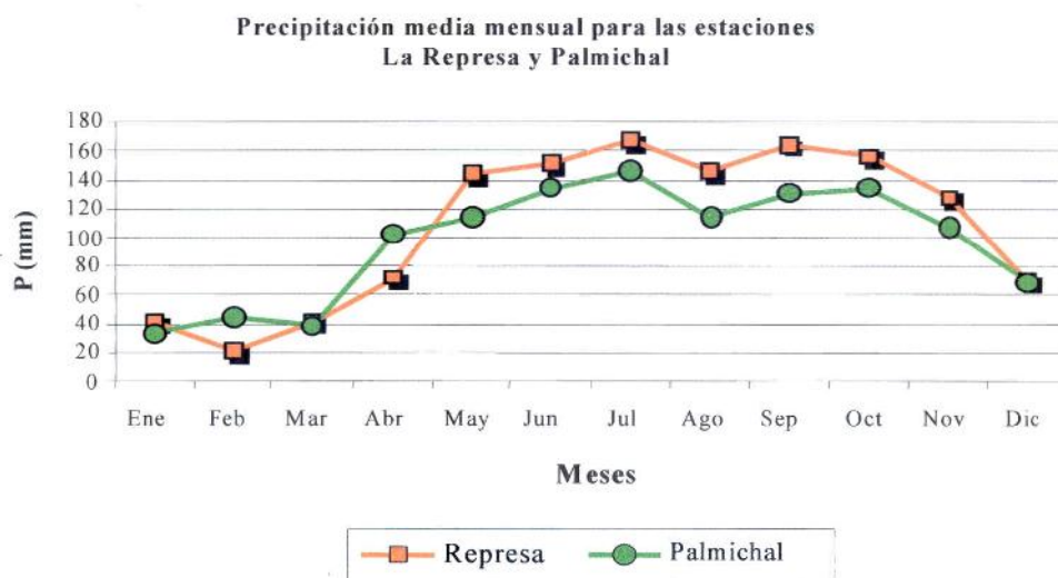
FIGURA 5. Precipitación media mensual para las estaciones La Represa y Palmichal.
