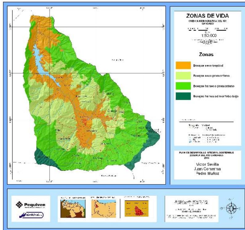
FIGURA 7. Mapa de zonas de vida según Holdridge.
