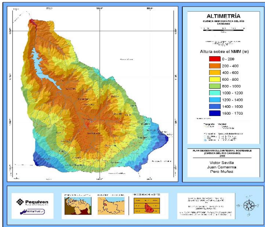
FIGURA 2. Modelo digital de elevación (MDE).
